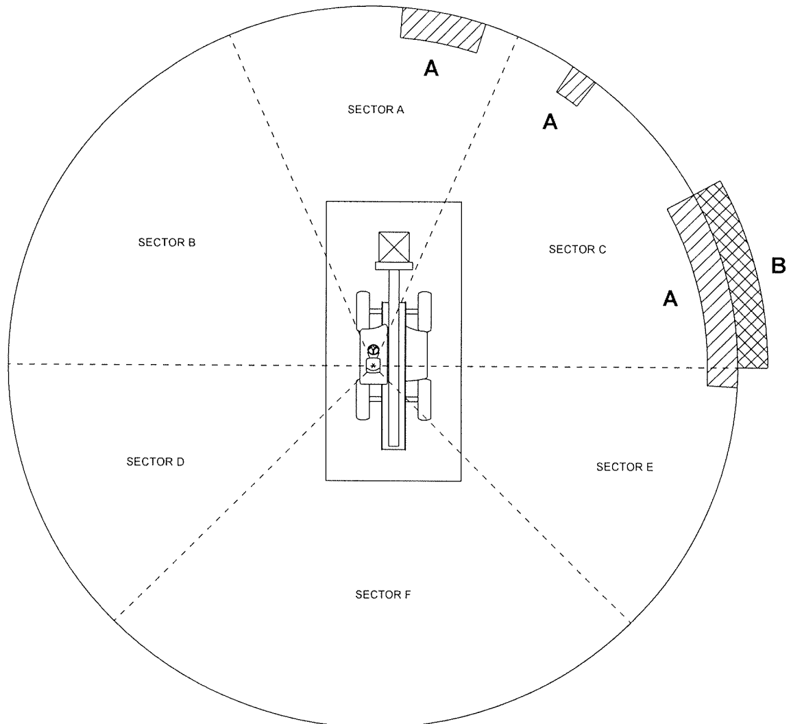
Figura 306. Obstrução à visibilidade em condição de carga suspensa
