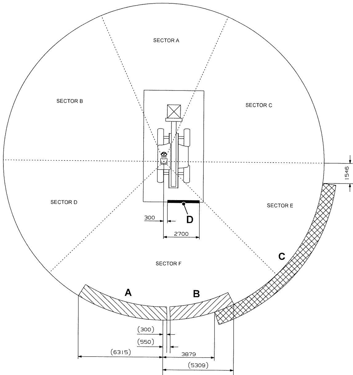
Figura 299. Configuração do espelho
