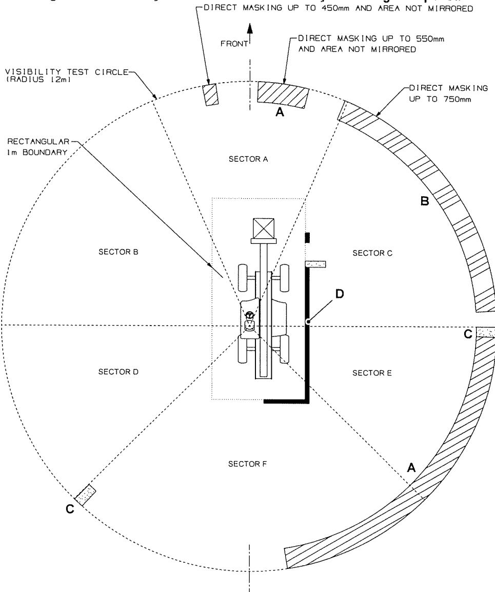
Figura 315. Obstrução à visibilidade em condição de carga suspensa
