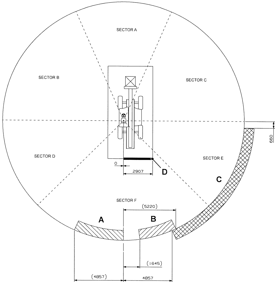
Figura 305. Configuração do espelho
