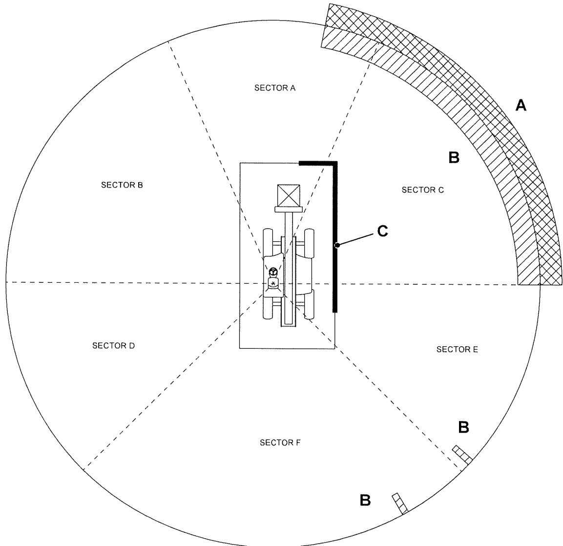
Figura 313. Obstrução à visibilidade em condição de carga de atrelado de camião
