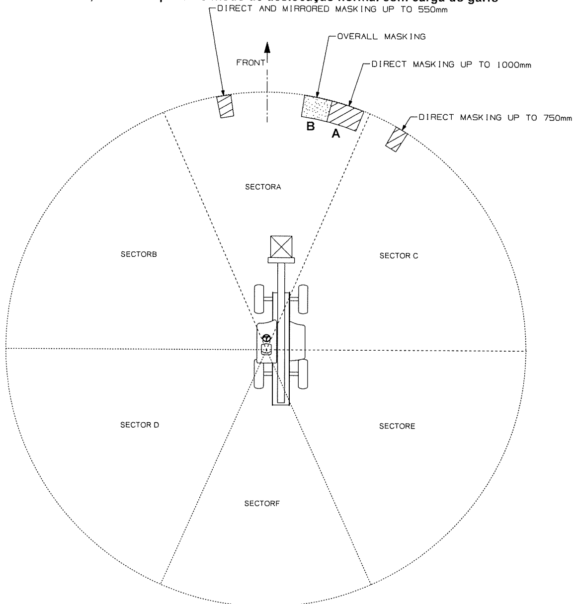
Figura 318. Obstrução à visibilidade nos setores A e C a um raio de 12 m, com a máquina no modo de deslocação normal com carga do garfo
