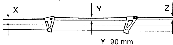
Figura 242. 3 correias
