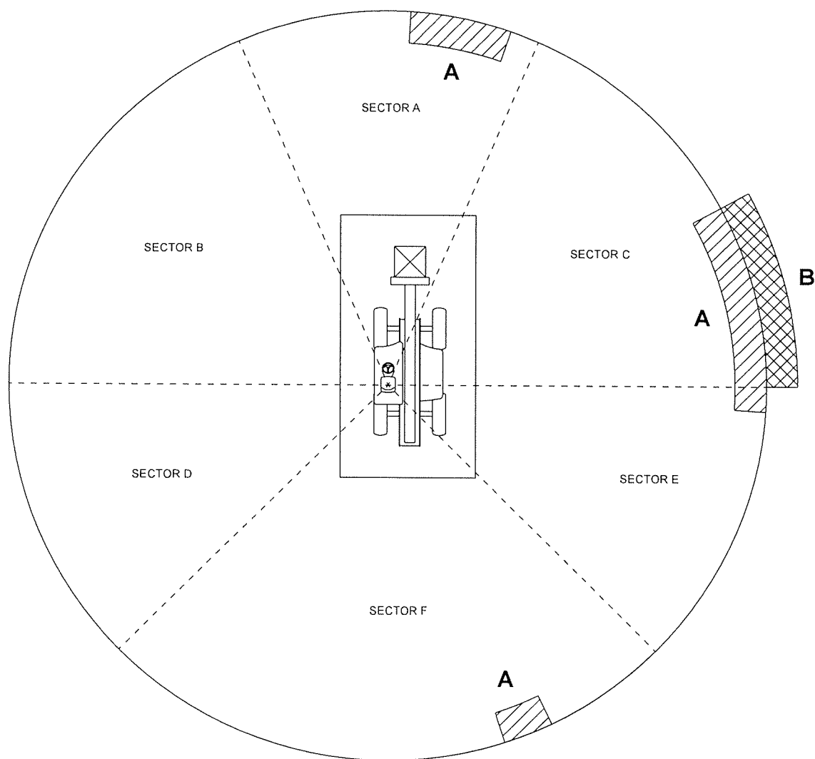
Figura 312. Obstrução à visibilidade em condição de carga suspensa
