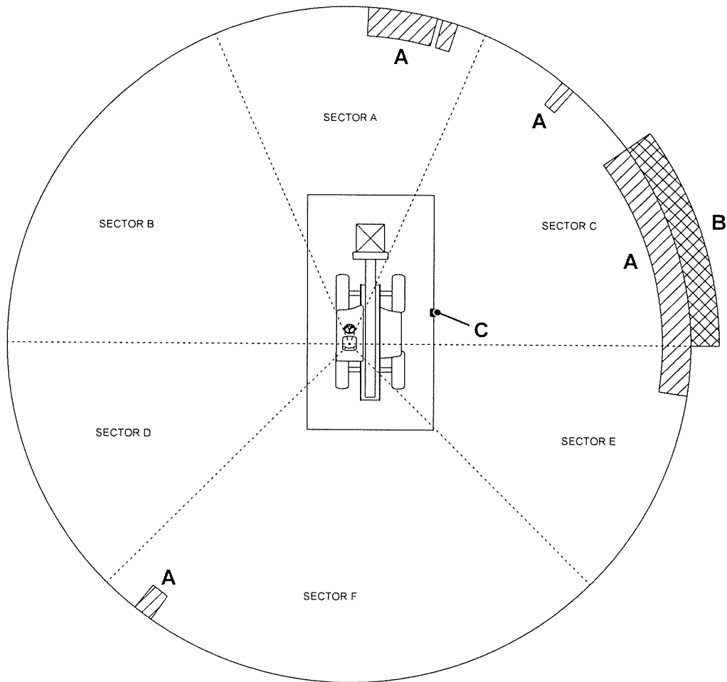
Figura 303. Obstrução à visibilidade em condição de carga suspensa
