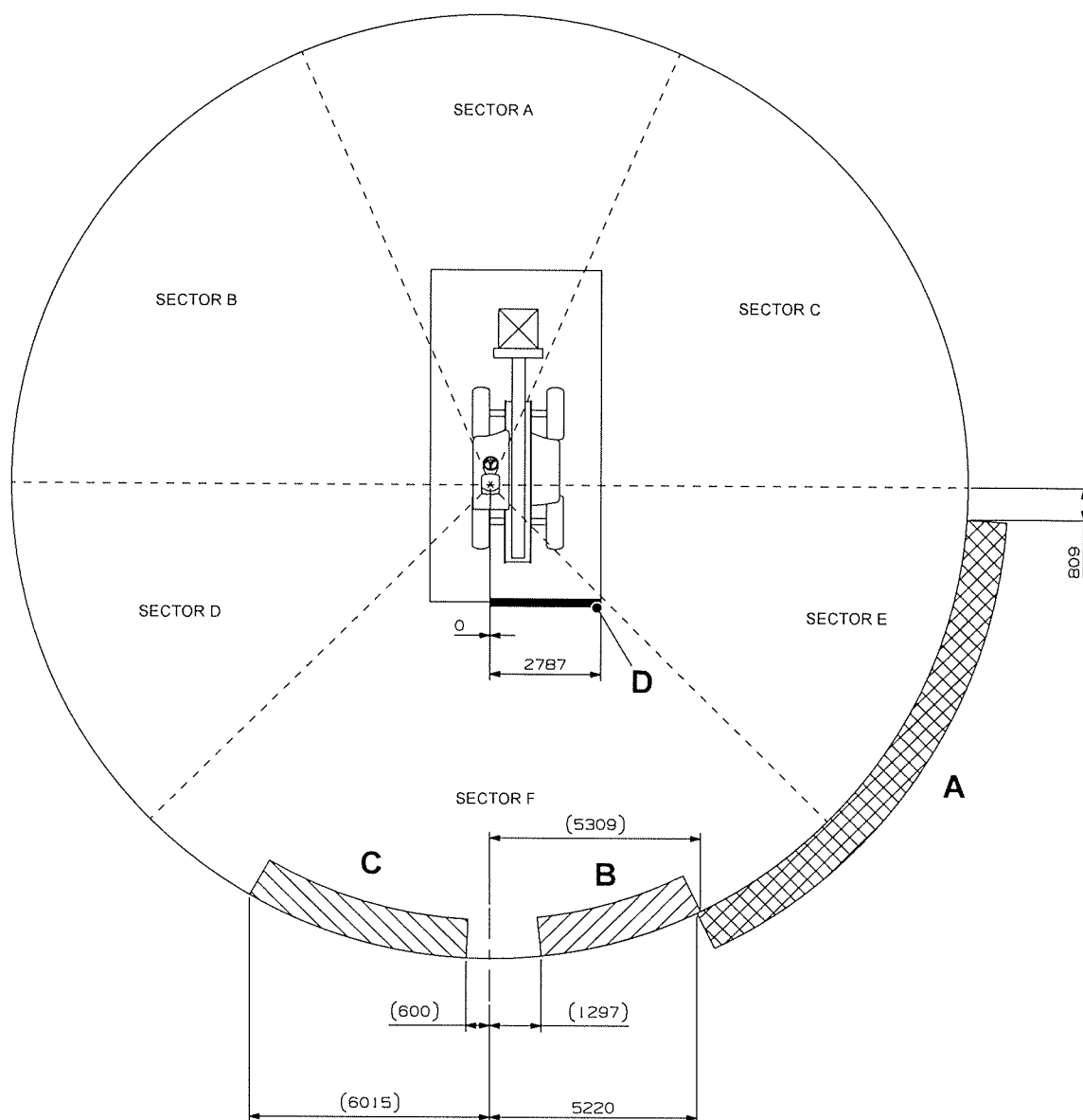
Figura 311. Configuração do espelho
