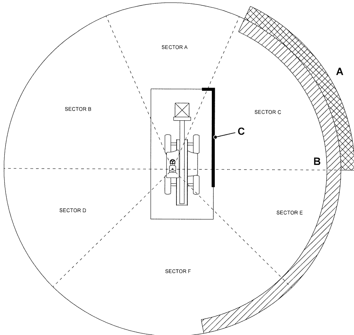
Figura 310. Obstrução à visibilidade em condição de carga de atrelado de camião
