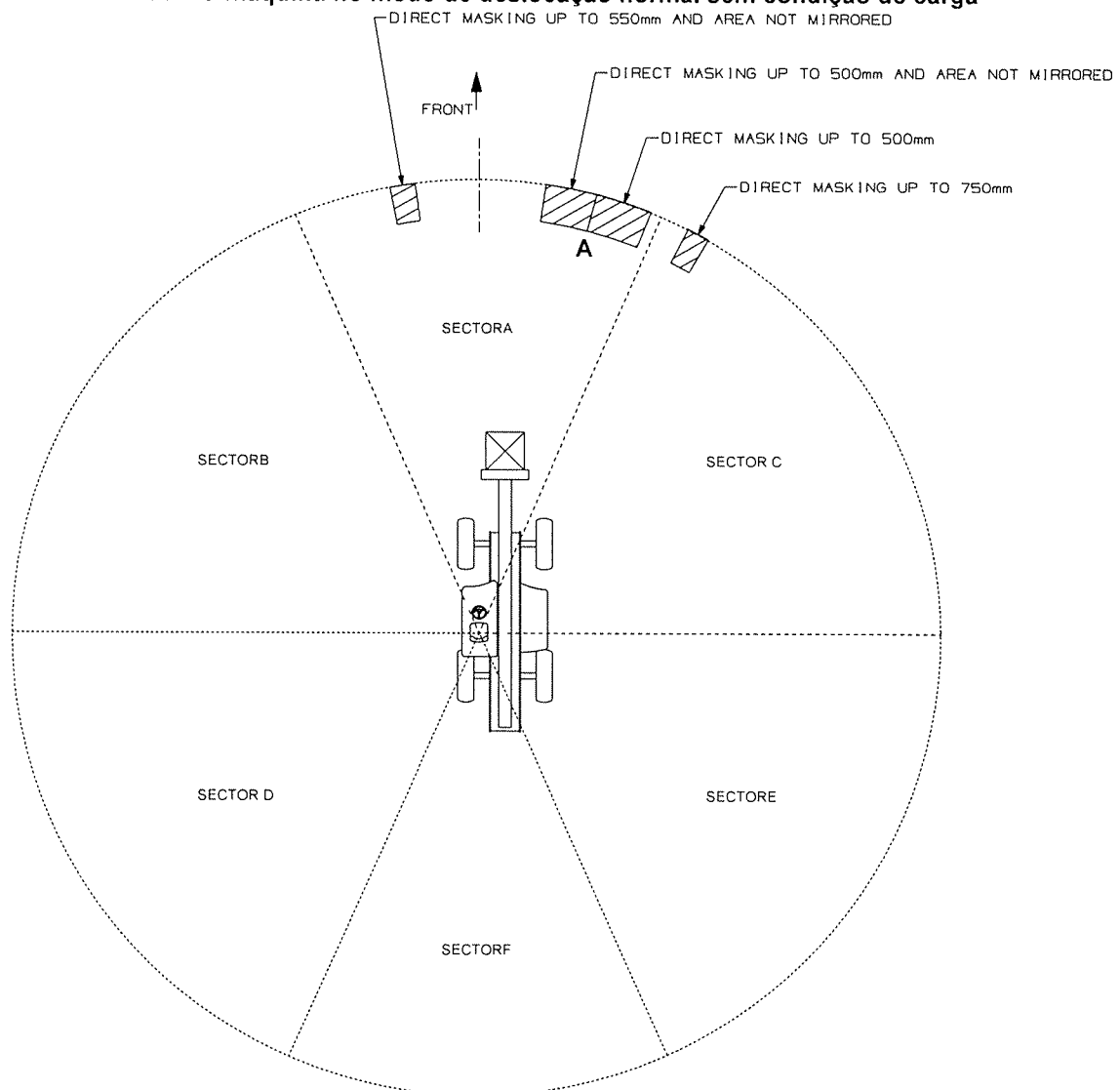
Figura 317. Obstrução à visibilidade nos setores A e C a um raio de 12 m, com a máquina no modo de deslocação normal sem condição de carga
