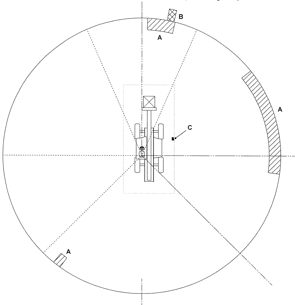
Figura 320. Obstrução à visibilidade em condição de carga suspensa
