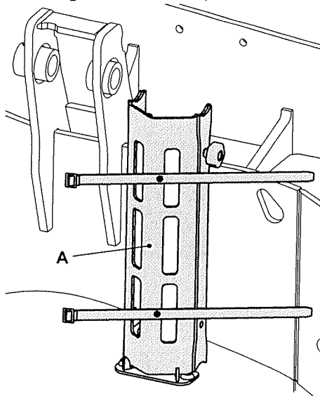
Figura 193. 508-66, 540-200
