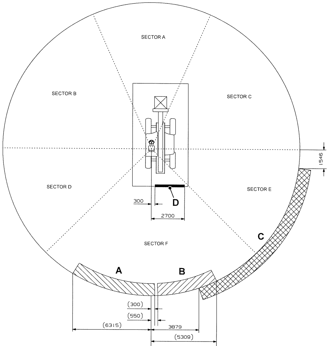
Figura 302. Configuração do espelho
