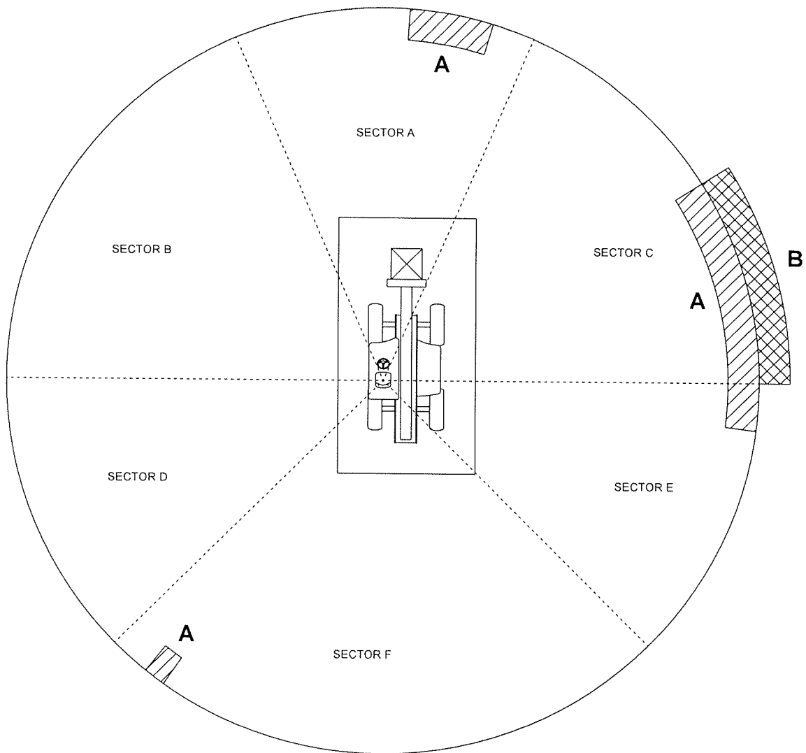
Figura 300. Obstrução à visibilidade em condição de carga suspensa
