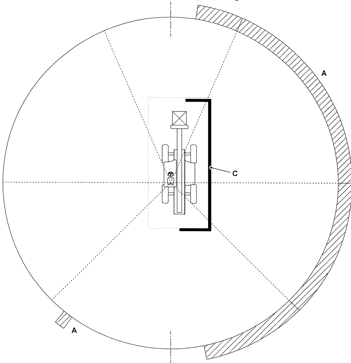
Figura 321. Obstrução à visibilidade em condição de carga de atrelado de camião
