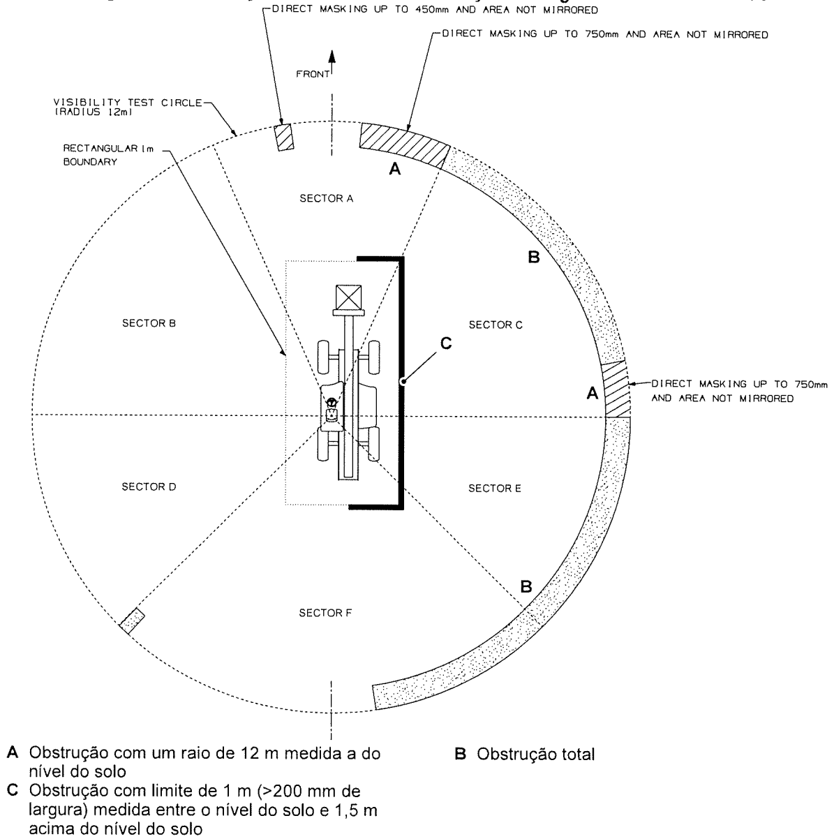
Figura 316. Obstrução à visibilidade em condição de carga de atrelado de camião
