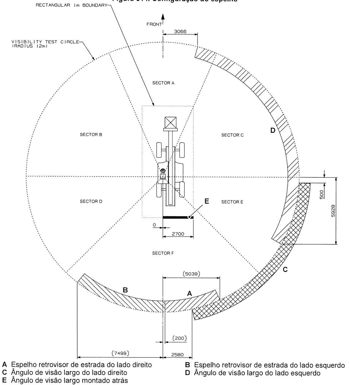
Figura 314. Configuração do espelho
