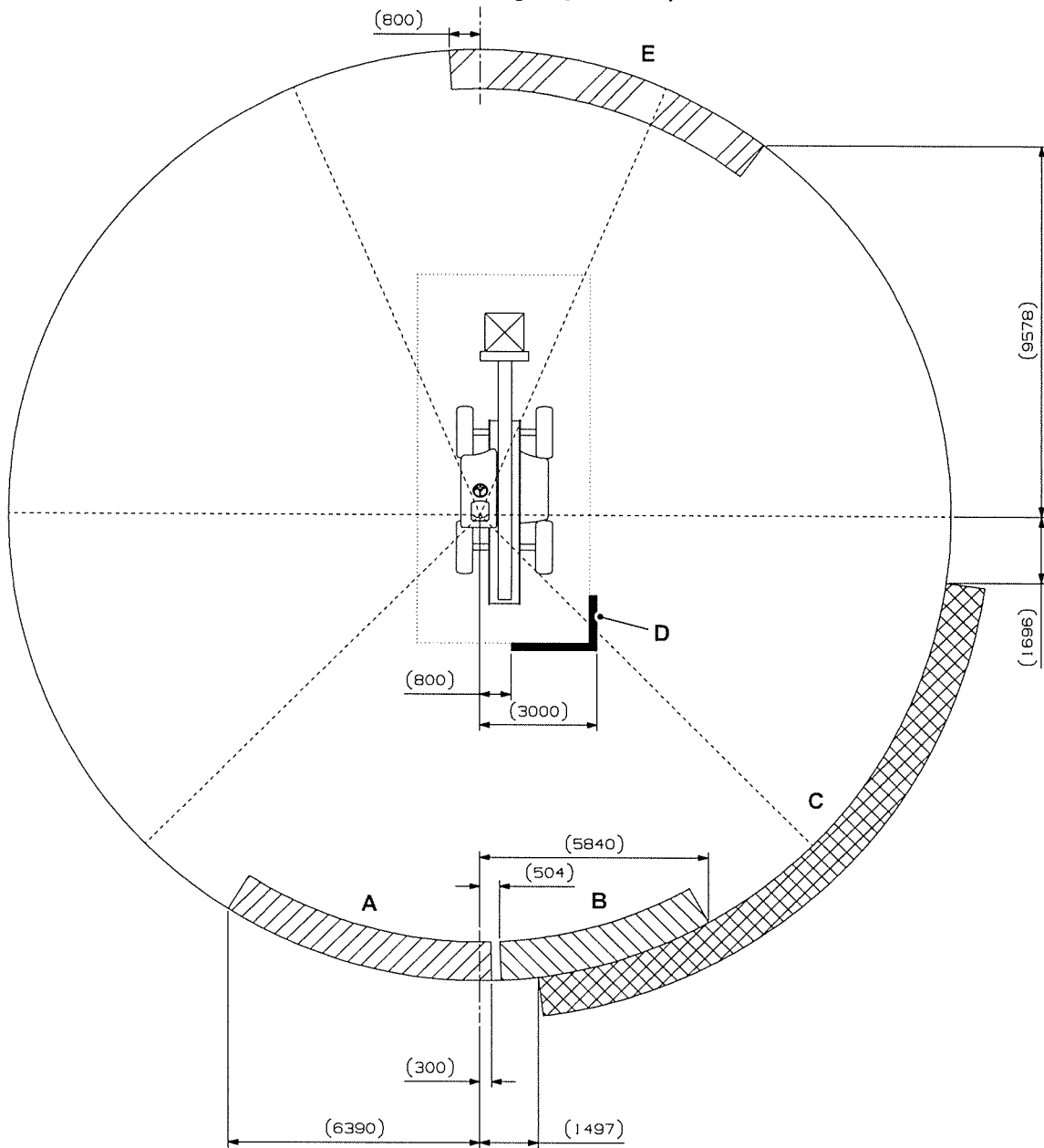
Figura 319. Configuração do espelho
