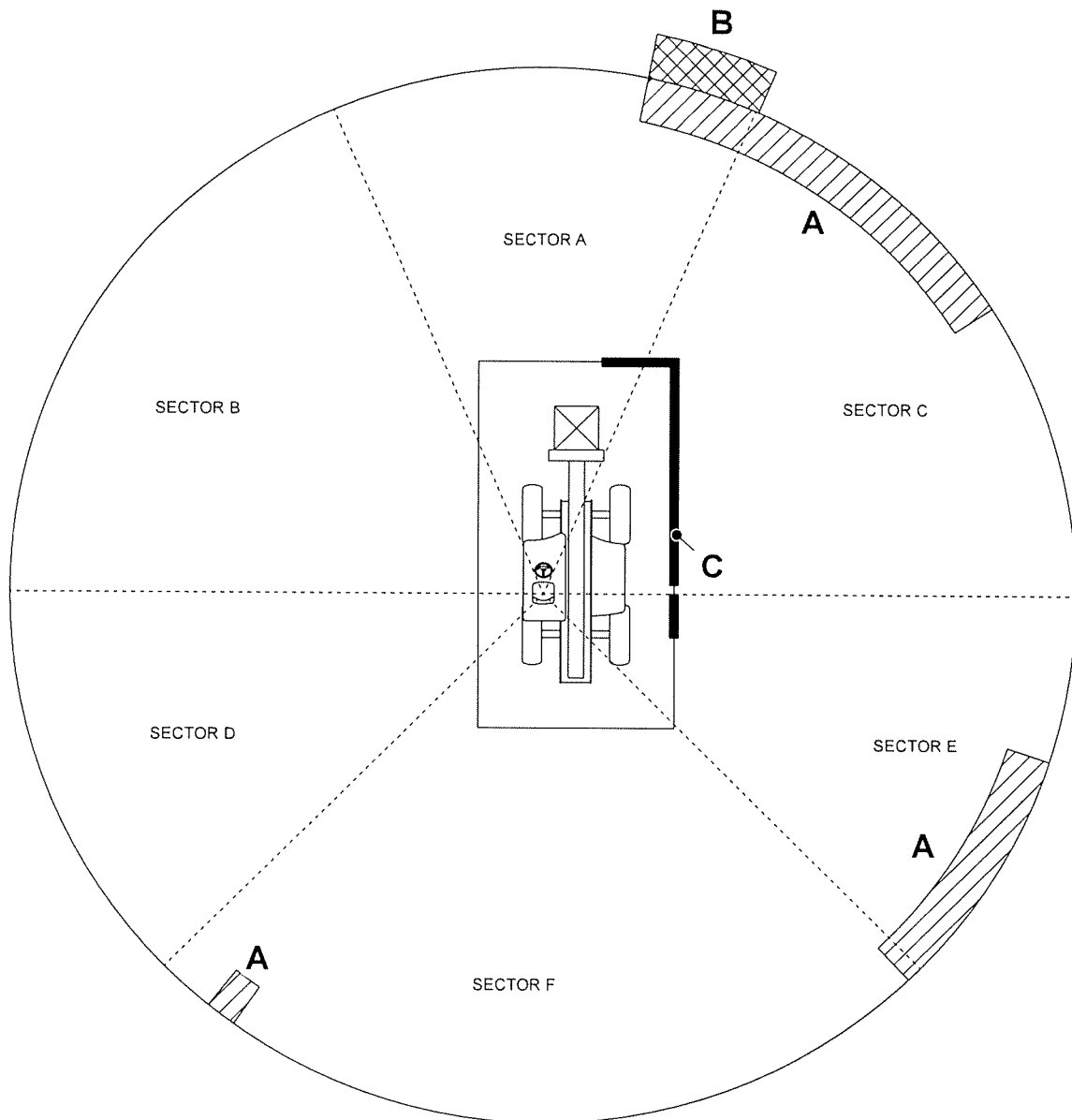
Figura 304. Obstrução à visibilidade em condição de carga de atrelado de camião
