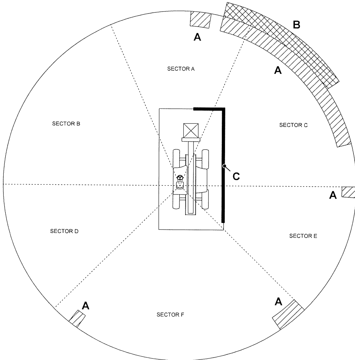
Figura 301. Obstrução à visibilidade em condição de carga de atrelado de camião
