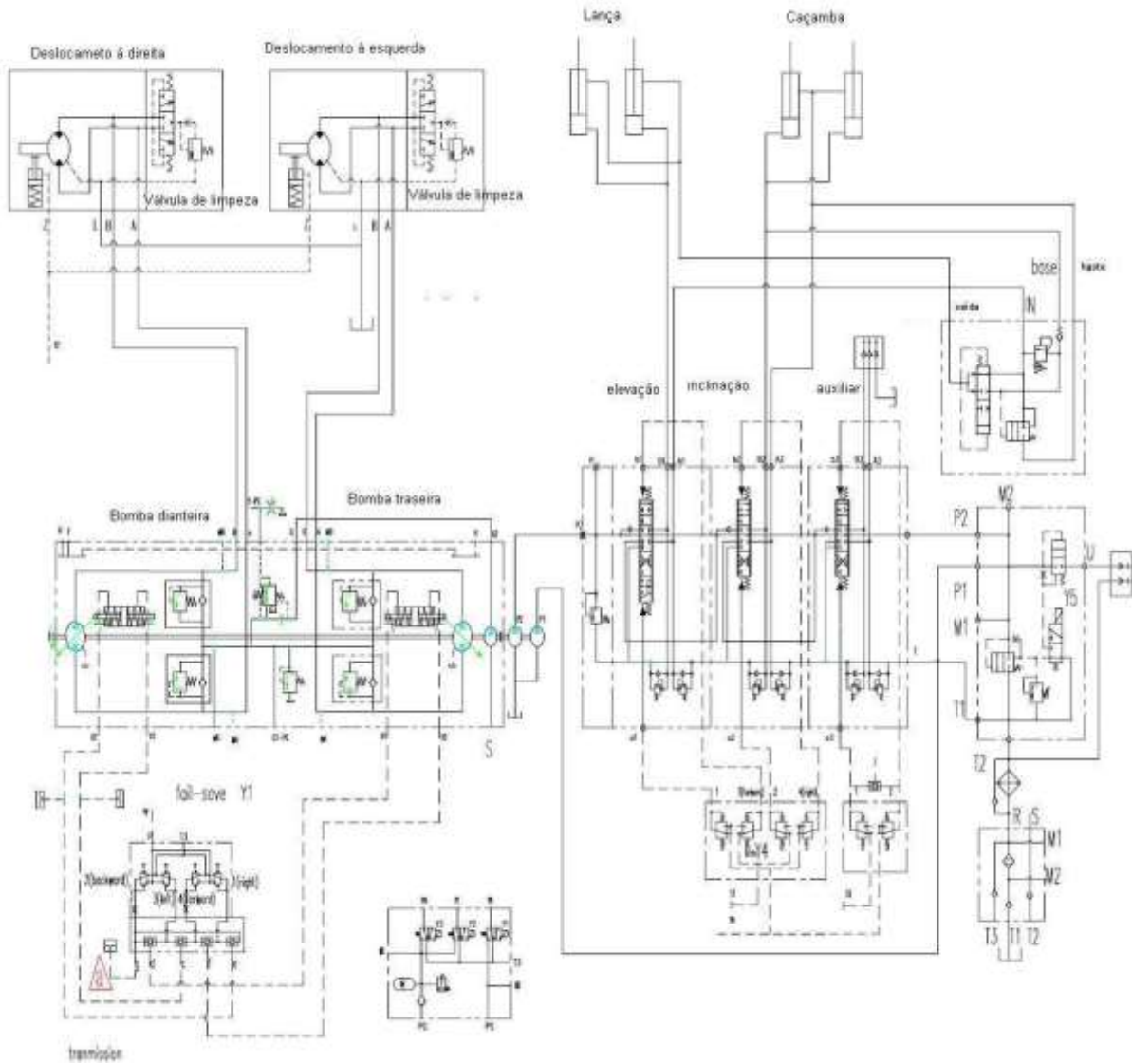
Diagrama Hidráulico da SWL3220 com Dispositivo de Alta Vazão (Opcional)
