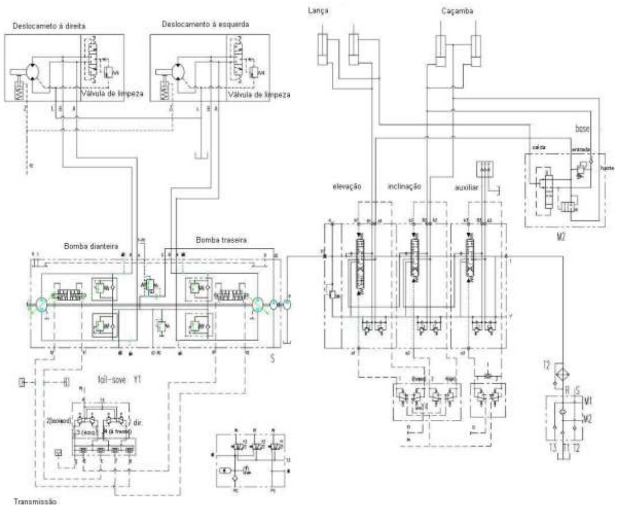
Diagrama Hidráulico da SWL3220
