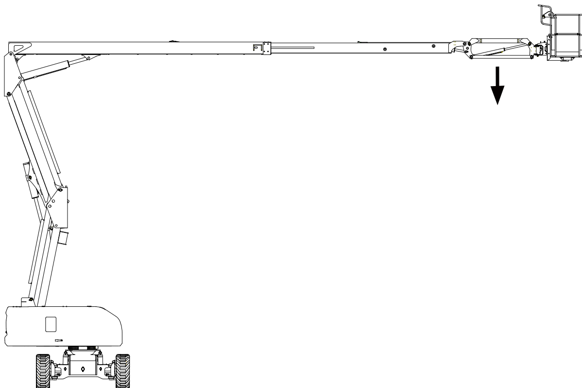
Fig. 2 Posição da menor estabilidade na frente da máquina
