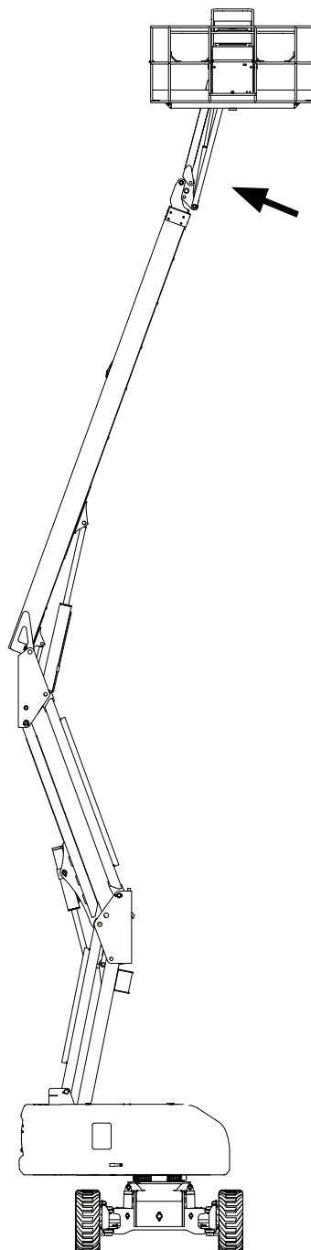
Fig. 3 Posição da menor estabilidade na traseira da máquina
