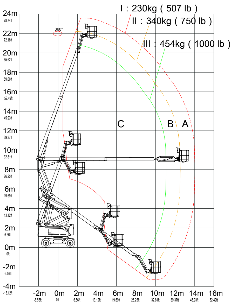
Fig. 1 Diagrama da área de trabalho (-5°)
