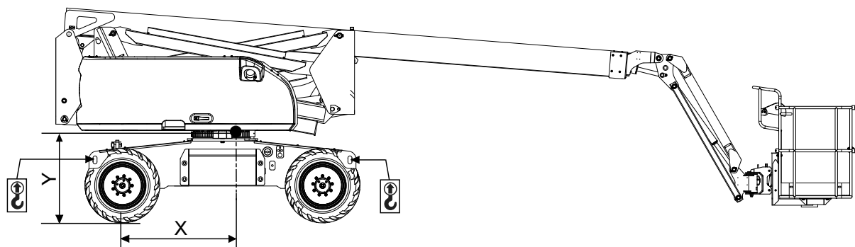
Fig. 11 Centro de gravidade e diagrama de elevação
